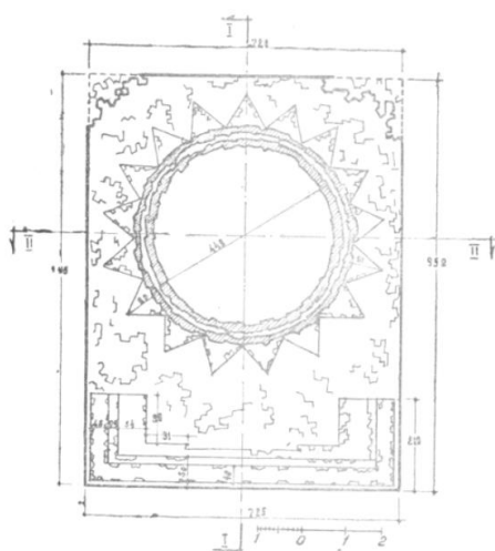
Рис. 32. Мавзолей Джоши-хан. План подкупольного барабана.
