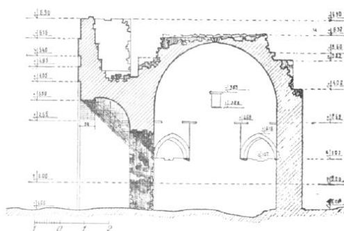
Рис. 35. Мавзолей Джоши-хан. Продольный разрез.
