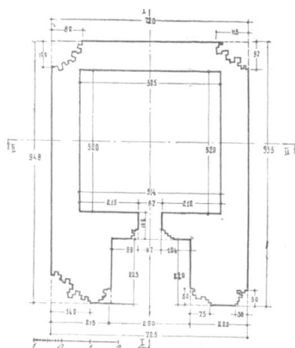
Рис. 33. Мавзолей Джоши-хан. План на отметке \pm 0,00 .
