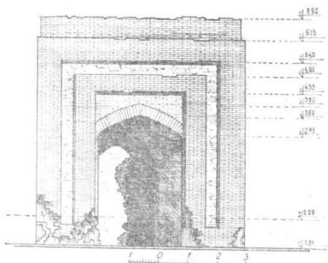
Рис. 31. Мавзолей Джоши-хан. Главный фасад.
