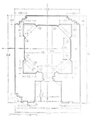
Рис. 34. Мавзолей Джоши-хан. План на отметке + 1,10.
